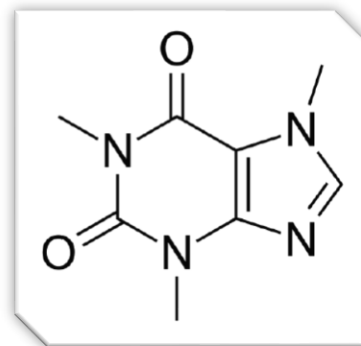
カフェインの分子構造
